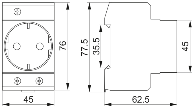
Габариты и размеры розетка на дин рейку
