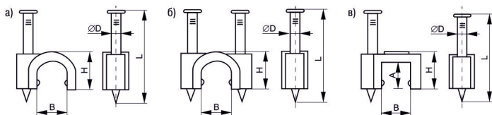
Рисунок 1. Габаритные размеры скоб: а) СКК4...СКК25, б) СКК30, СКК35, в) СКП
